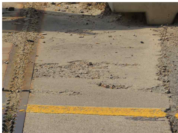
A1 신축이음 후타재박락 (0.3m×0.3m)
