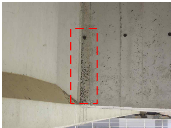
가로보 S2-G3~G4-CB6 재료분리 (0.2m×1.0m)
