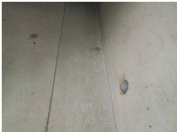
가로보 S11-G4~G5-CB7 균열 (0.3mm/0.5m)
