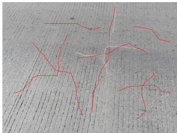
S2 교면포장 망상균열 ( 2.5\text{m} \times 7.0\text{m} )
