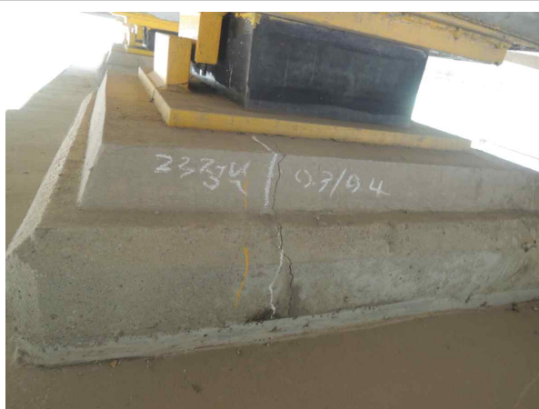
P1-SH3 받침물탈균열 (0.3mm/0.4m)
