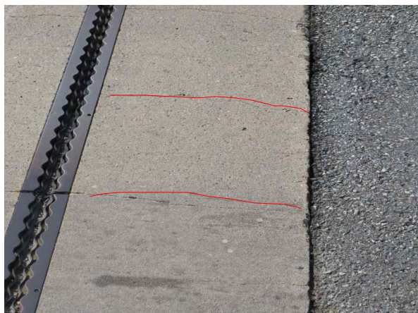
A1 신축이음 후타재균열 (0.1mm/0.5m, 31EA)
