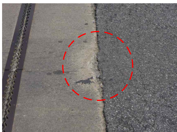
A2 신축이음 후타재파손 (0.1m×0.3m)
