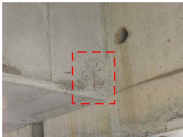
가로보 S6-G1~G2-CB1 철근노출 및 박락 (0.2m×0.2m)
