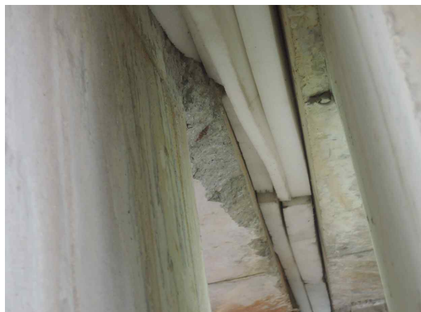
S12 바닥판 하면 철근노출 및 박락(2.3m×0.3m)
