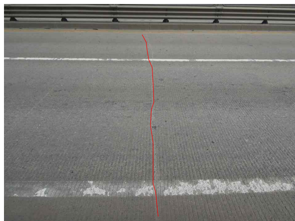
S13 교면포장 균열 ( L=6.0\text{m} )
