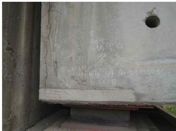
거더 S14-G1 보수부박락 (0.2m×1.8m)
