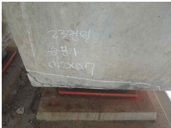
거더 S9-G7 층분리 (0.2m×0.7m)
