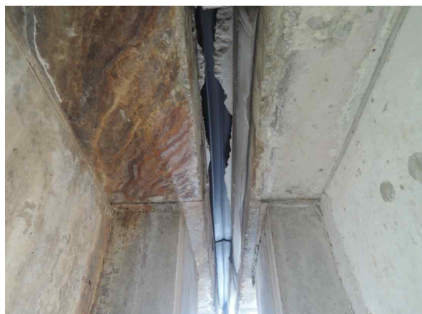
P9 신축이음 하부 누수 (L=4.0m)
