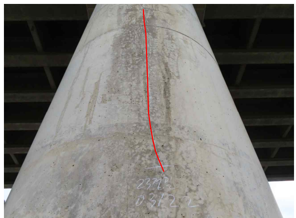
P12 교각 균열 (0.3mm/2.2m)
