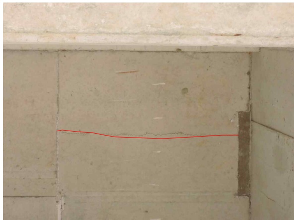
S3 바닥판 하면 균열(0.3mm/1.0m)
